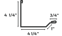
DOOR EDGE
