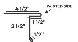
DRIP EDGE
