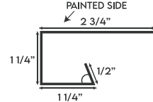
JAMB TRIM
